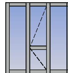
Cloison fixe avec porte
